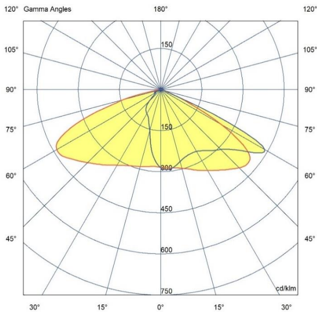
СВЕТЛОРАЗПРЕДЕЛИТЕЛНА ДИАГРАМА
